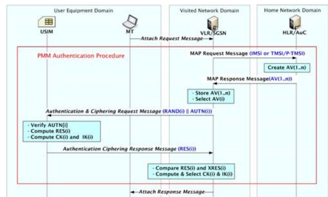
Fig. 2. UMTS-AKA procedure
